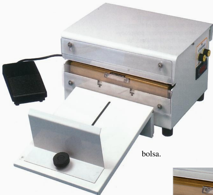
Codificador
