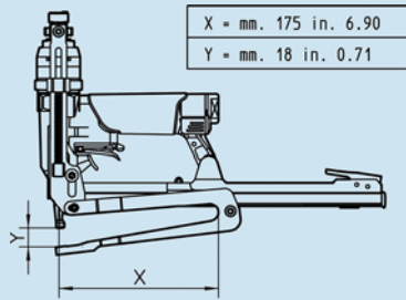
1B 50-16 Carton Plier
