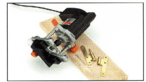
Detalle cabezal pernios.
