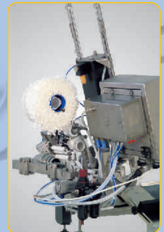
Loop inserter GSA25
